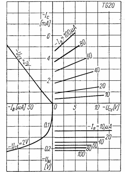
Rys. 23. Charakterystyki statyczne tranzystora TG20
