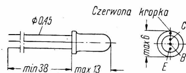
Rys. 21. Główne wymiary tranzystorów TG10 i TG20
