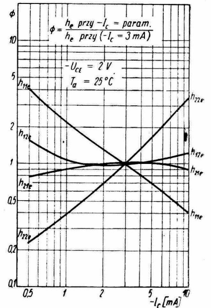
Rys. 8. Zależność parametrów h_e od prądu kolektora I_C
