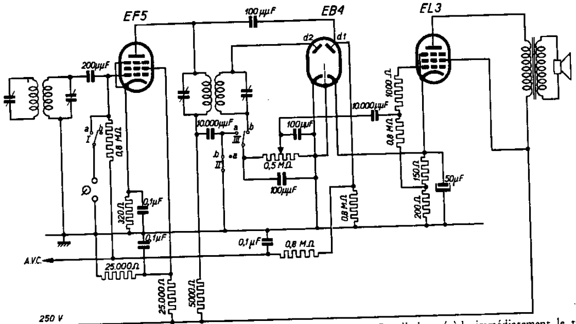
Montage de la partie M.F. et B.F. d'un récepteur utilisant le tube EL 3. La diode précède immédiatement le tube de sortie; pour l'amplification phonographique, l'étage M.F. est utilisé comme préamplificateur. La commutation se fait comme l'indique la figure. Dans la position „a” des commutateurs I, II et III le récepteur peut recevoir la tension du pick-up; dans la position „b” il assure la réception des émissions de radio.
