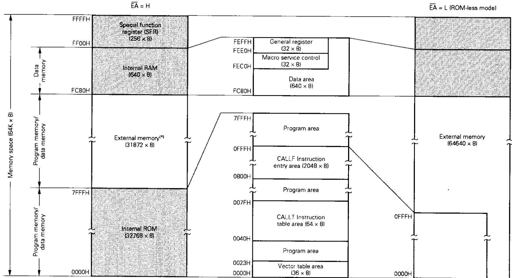
Fig. 2-3 Memory Map (μPD78138)
