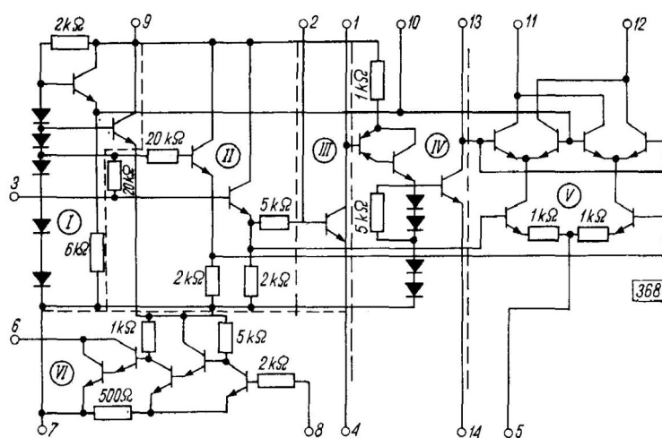
Schemat elektryczny
