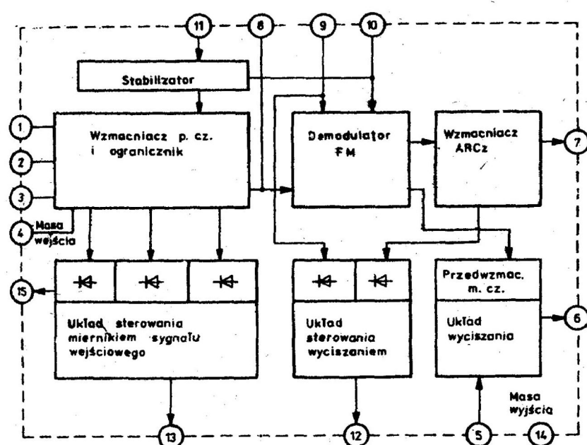
Schemat blokowy
