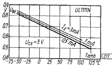
Napięcie baza-emiter w funkcji temperatury otoczenia
