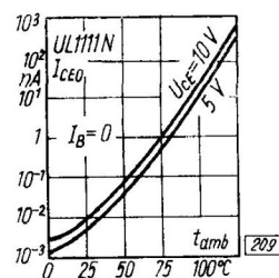
Prąd zerowy kolektor-emiter w funkcji temperatury otoczenia
