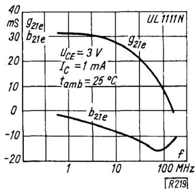
Admitancja przejściowa w funkcji częstotliwości
