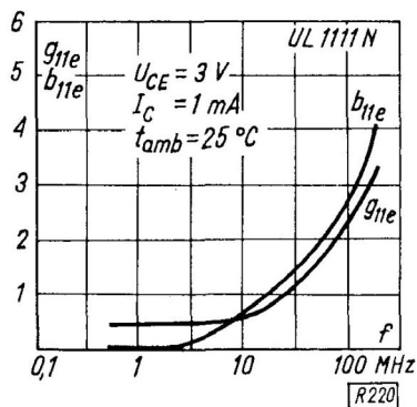
Admitancja wejściowa w funk- cji częstotliwości
