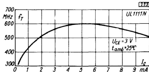
Zależność częstotliwości gra- nicznej w funkcji prądu ko- lektora
