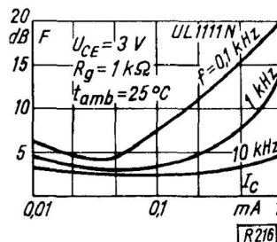
Współczynnik szumów w funkcji prądu kolektora ( R_g = 1 k\Omega )
