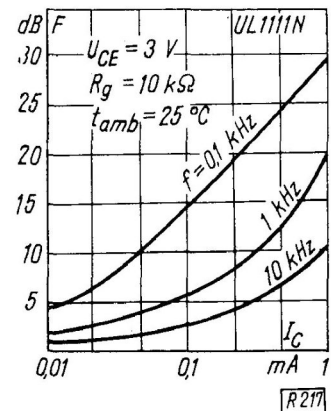
Współczynnik szumów w funkcji prądu kolektora ( R_g = 10 k\Omega )
