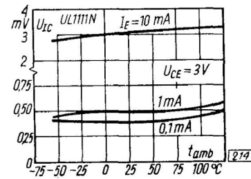
Napięcie wejściowe niezrównoważenia w funkcji temperatury otoczenia
