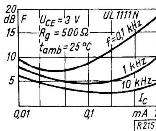
Współczynnik szumów w funkcji prądu kolektora ( R_g = 500 \Omega )
