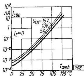
Prąd zerowy kolektor-baza w funkcji temperatury otoczenia
