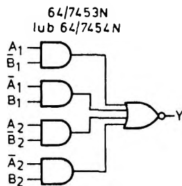
Rys. 2.98. Zastosowanie bramki I-LUB-NIE w układzie dwupozycyjnego komparatora A = B
