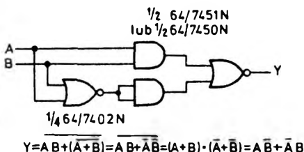
Rys. 2.96 Układy realizujące funkcję WYŁĄCZNIK-LUB (EXCLUSIVE-OR)
