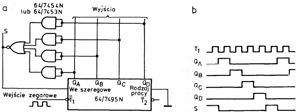
Rys. 2.104. Licznik pierścieniowy samokorygujący
