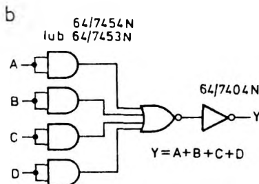
Rys. 2.92 Układy realizujące funkcję LUB
