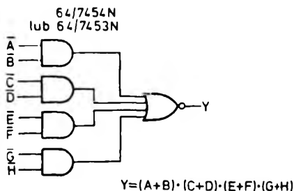
Rys. 2.95 Układy realizujące funkcję LUB-I
