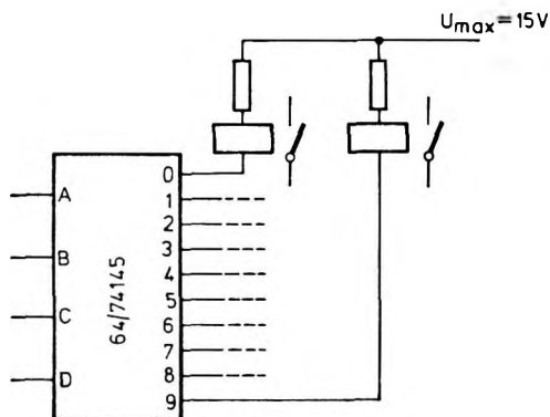
Rys. 3.49. Przykład zastosowania dekodera 64/74145 w układzie sterowania przełącznikami
