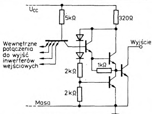
Schemat ideowy bramki wyjściowej
