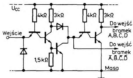
Schemat ideowy pary inwerterów wejściowych
