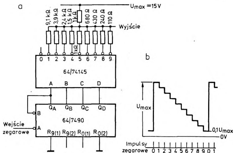
Rys. 3.50 Generacja przebiegów schodkowych a — schemat ideowy, b — przebieg wyjściowy
