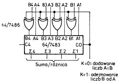
Rys. 3.95. Układ wykonujący operacje dodawania lub odejmowania
