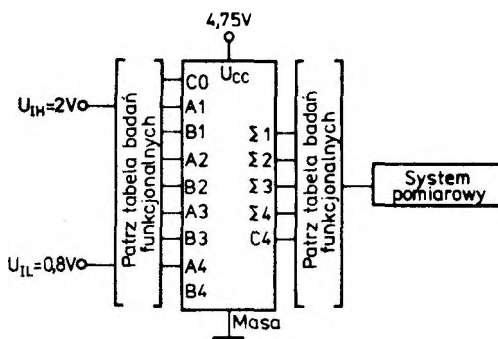
Układ badań funkcjonalnych
