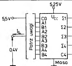
Układ pomiarowy D. Pomiar I_{IL}
