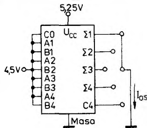
Układ pomiarowy F. Pomiar I_{OS}
