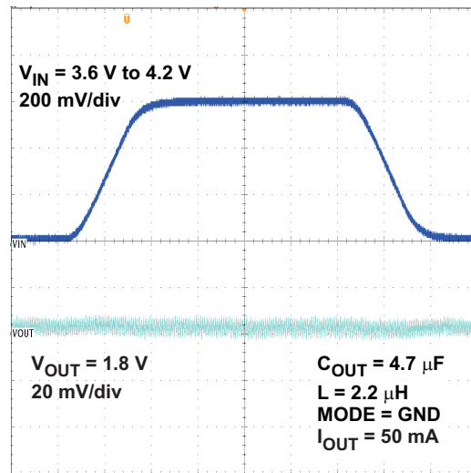
t - Time - 10 \mu\text{s} /div
