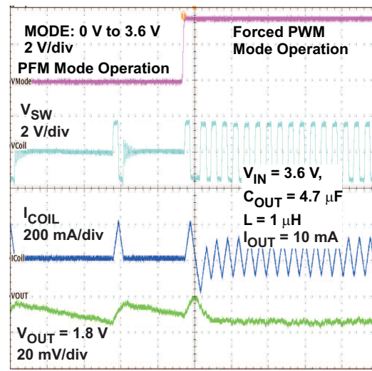
t - Time - 1 \mu\text{s} /div
