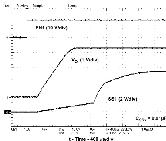
Figure 10. \text{VO1}=3.3\text{V} , SoftStart
