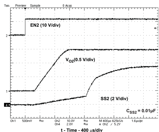
Figure 11. \text{VO2}=1.5\text{V} , SoftStart
