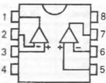
DIP8 SO8
