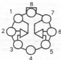
TO-99
