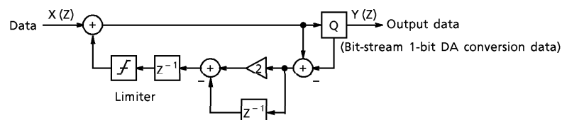
Fig.6. \Sigma - \Delta modulation DA converter
