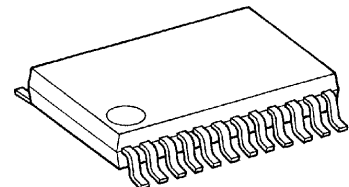
SSOP24-P-300-0.65A
