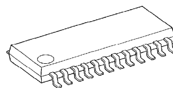
SSOP24-P-300-1.00B
