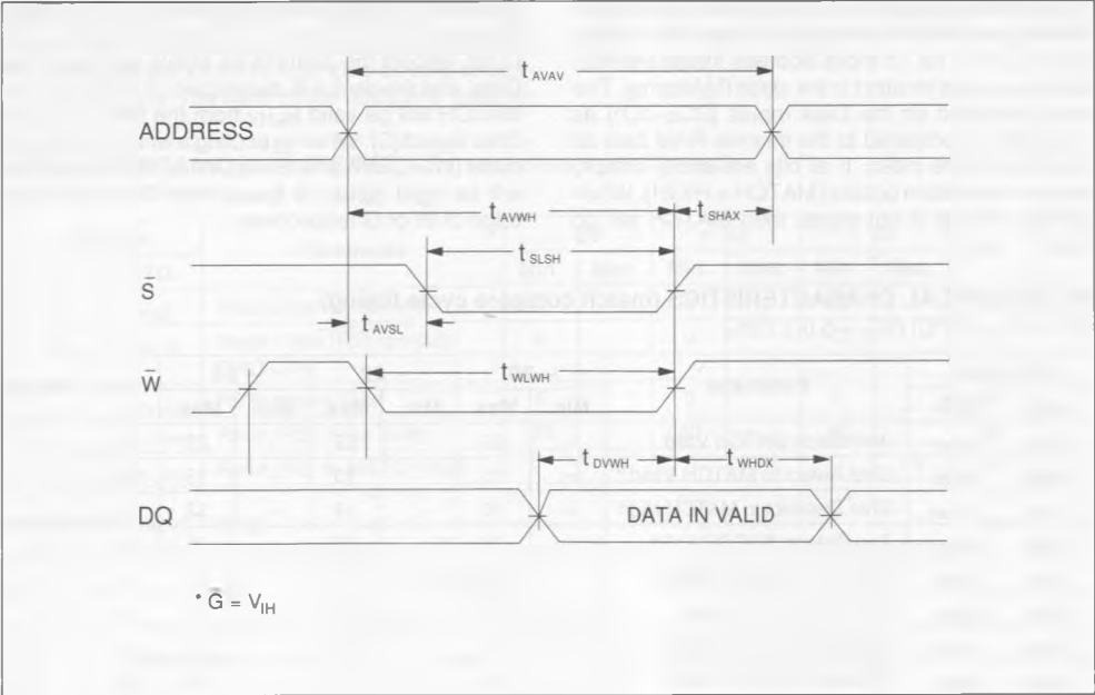
Figure 4b : Write Timing N°2 ( \overline{S} control).
