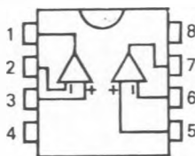
DIP8 SO8
