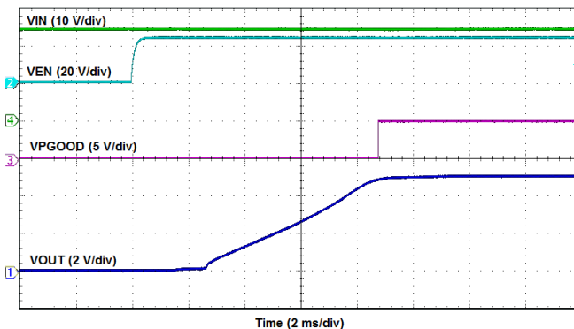
Figure 24. Enable Turn-ON
