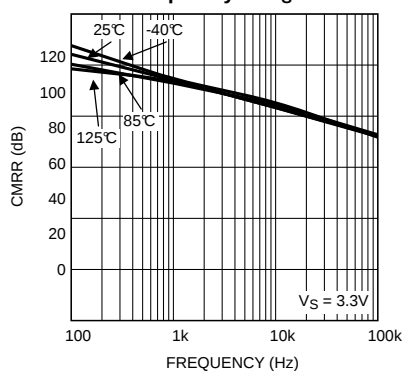
CMRR
