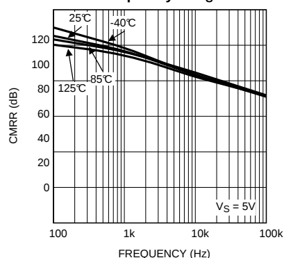
CMRR
