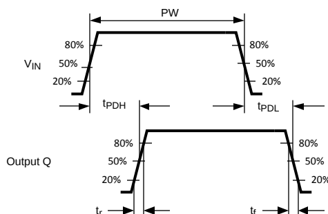
Figure 5. Pulse Parameter
