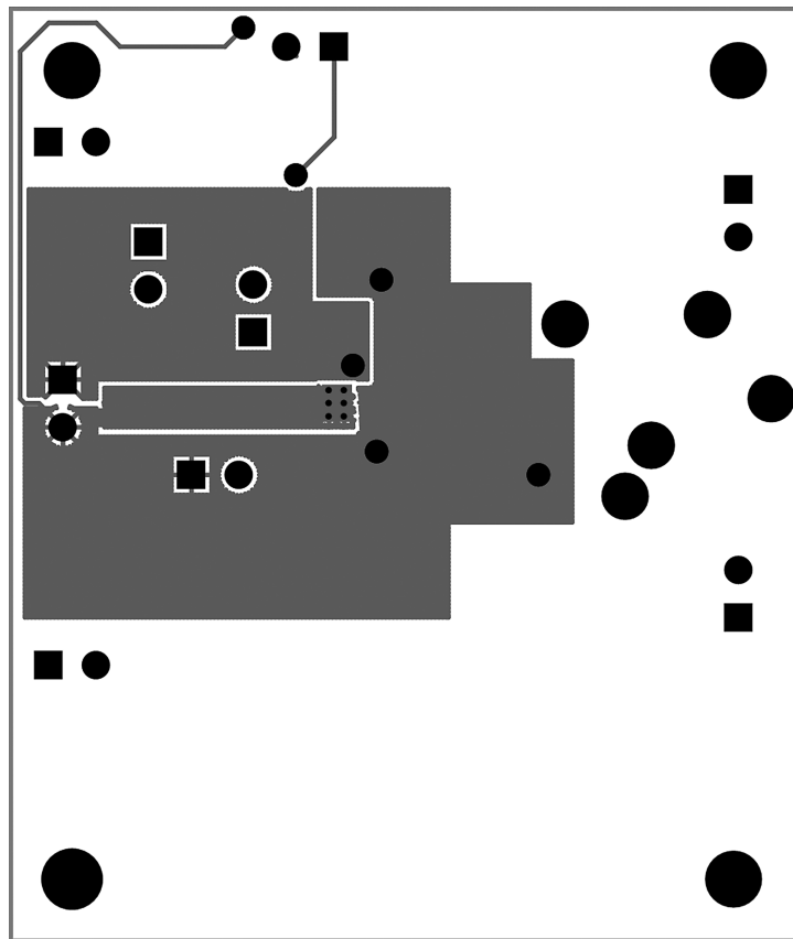
Figure 47. Bottom Layer
