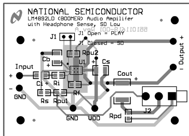
Top Layer
