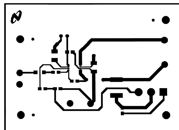
Bottom Layer
