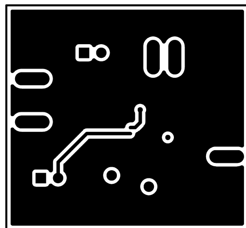
Figure 24. Bottom Layer
