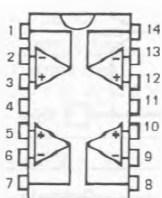
DIP14/CERDIP14 SO14
