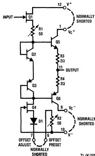
LH0033/LH0033A
