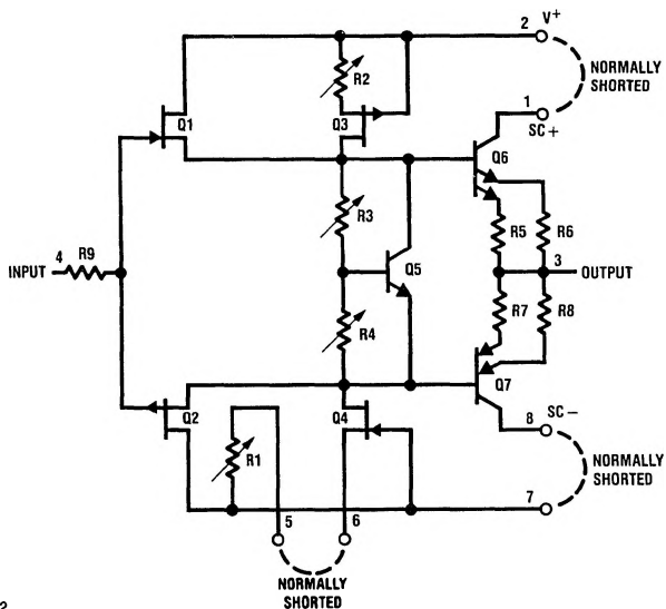
LH0063
