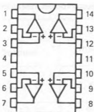
DIP14/CERDIP14 SO14
