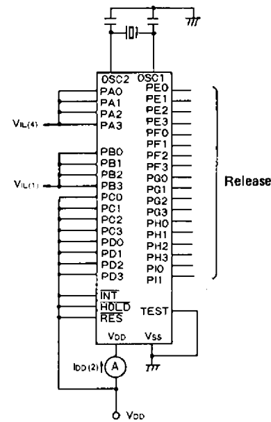
Fig. 3 I_{DD(2)} test circuit
