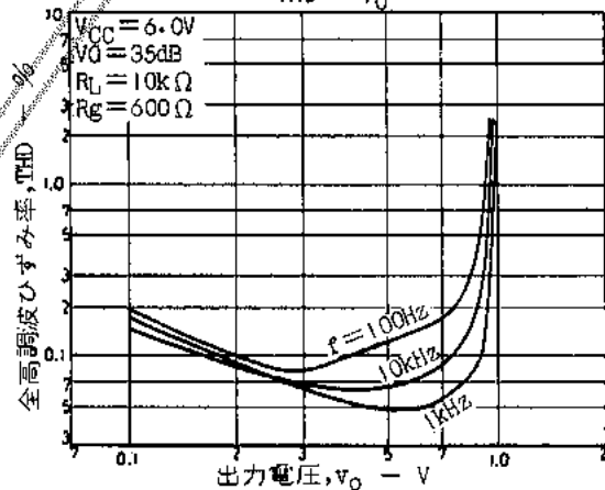
THD - V_O
