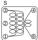
FM OSC (SA-1052)
