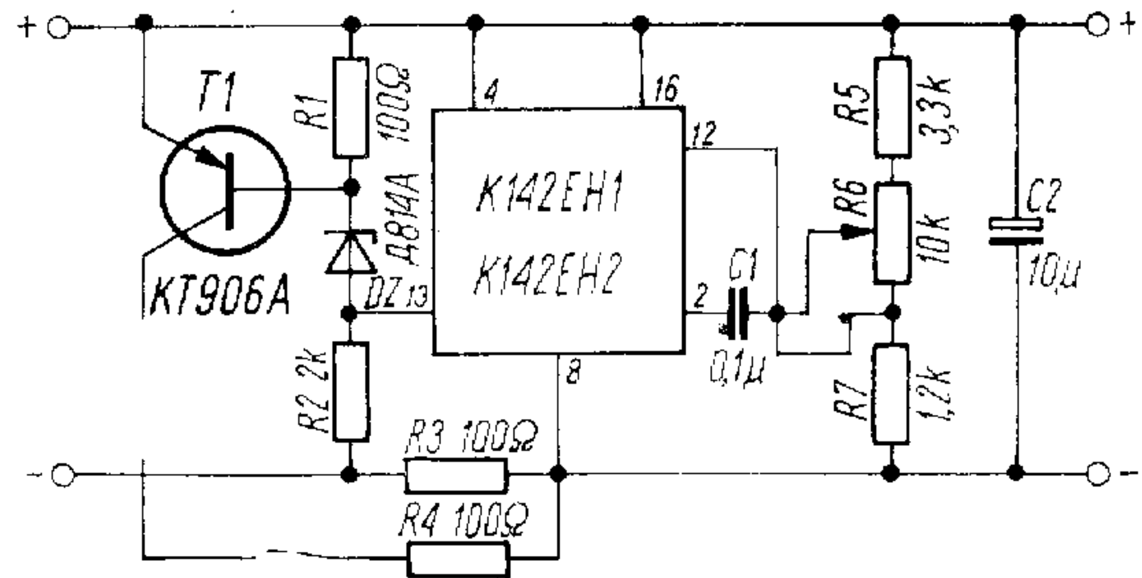
Rys. 19. Schemat układu stabilizatora równoległego
