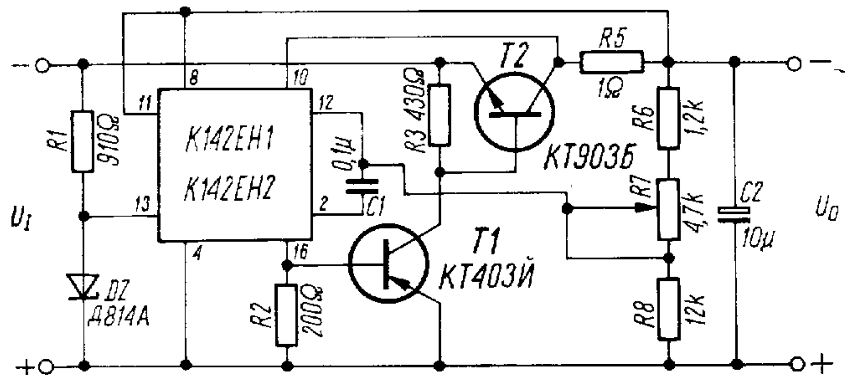
Rys. 20. Schemat układu stabilizatora ujemnego napięcia
