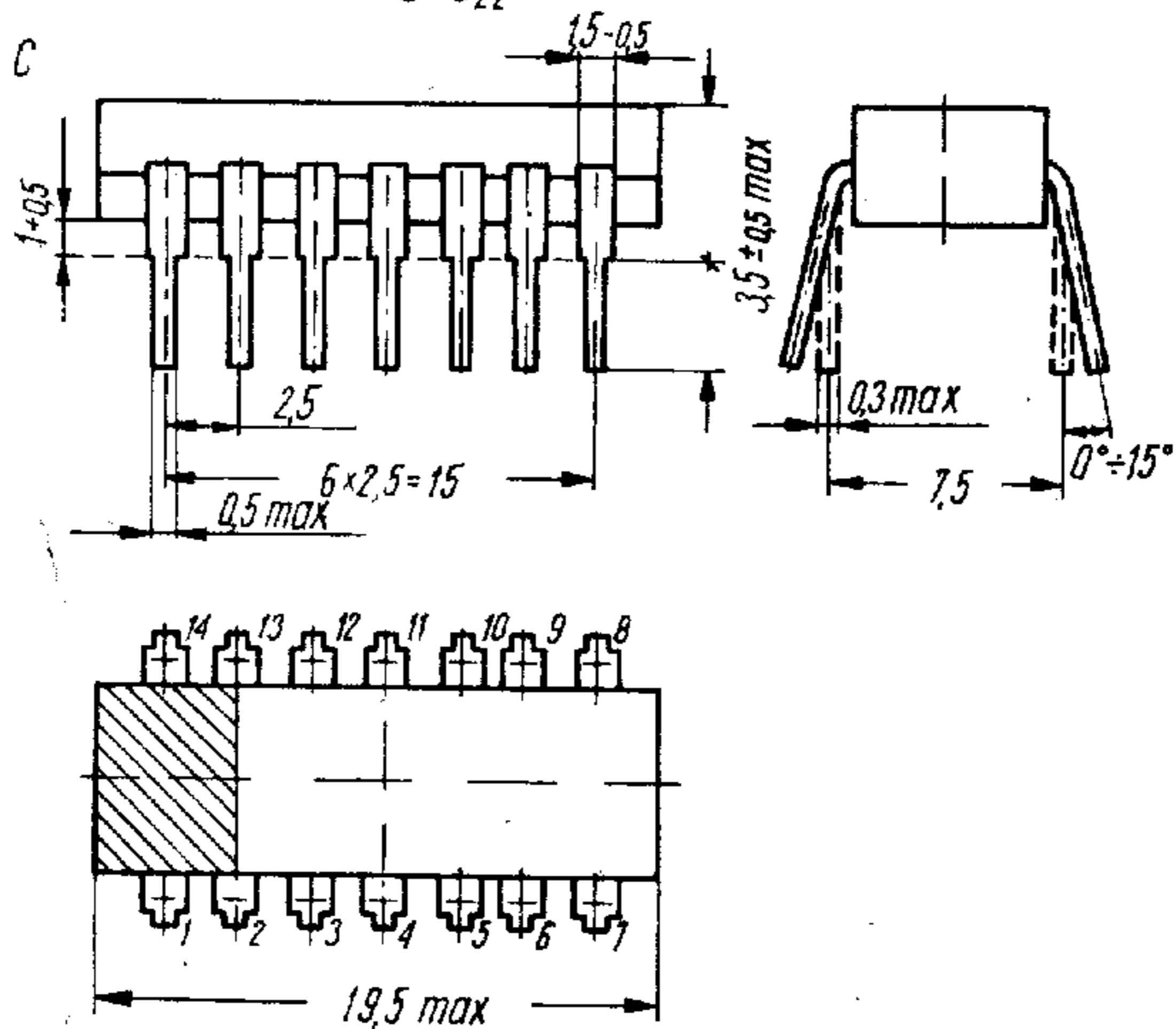
Rys. 1. Układ wzmacniacza różnicowego K118UD1 a – schemat, b – typowy układ pracy, c – szkic obudowy typu 201.14-6
