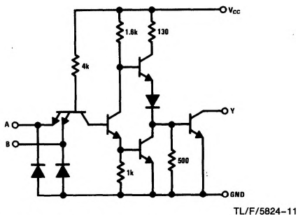
DS55451/DS75451
