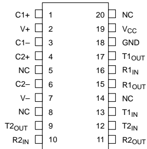
20-PIN TSSOP
