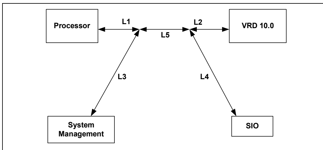
Figure 47. VID Topology
